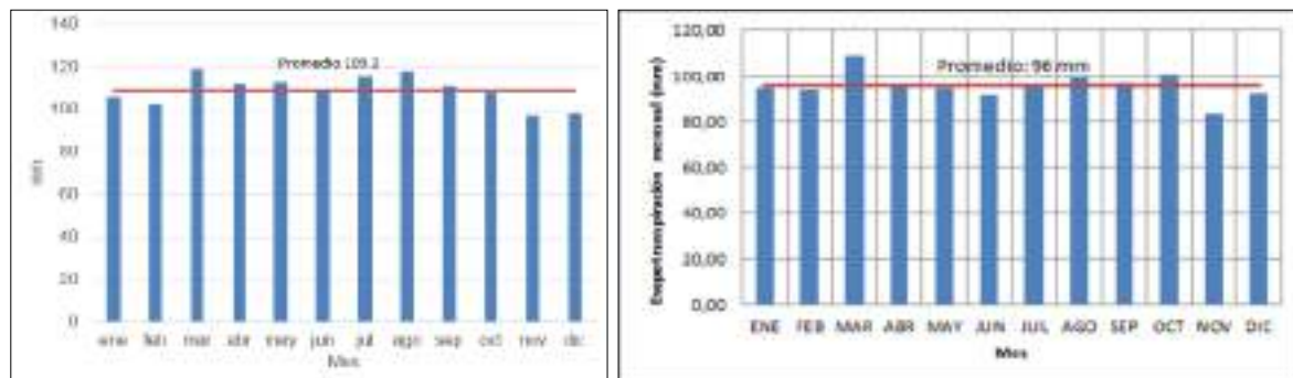
Figura 6-23 Evapotranspiración Potencial Estación Vivero Surata año 1992, condición Niño Método Hargreaves (izquierda) Método Penman (derecha)
